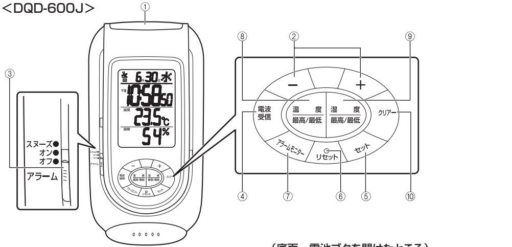
(底面 電池ボタンを開けたところ)
