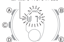
磁気偏角の方角と角度
