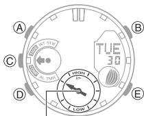
潮の干満 (タイドグラフ)
