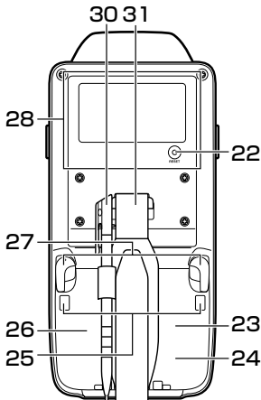
<裏面>
