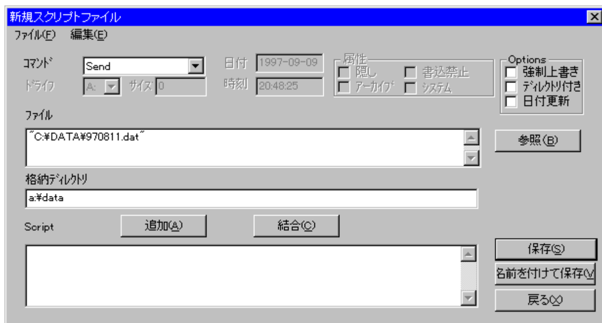
図4-3. LMWINのSCRIPTファイル新規作成画面
