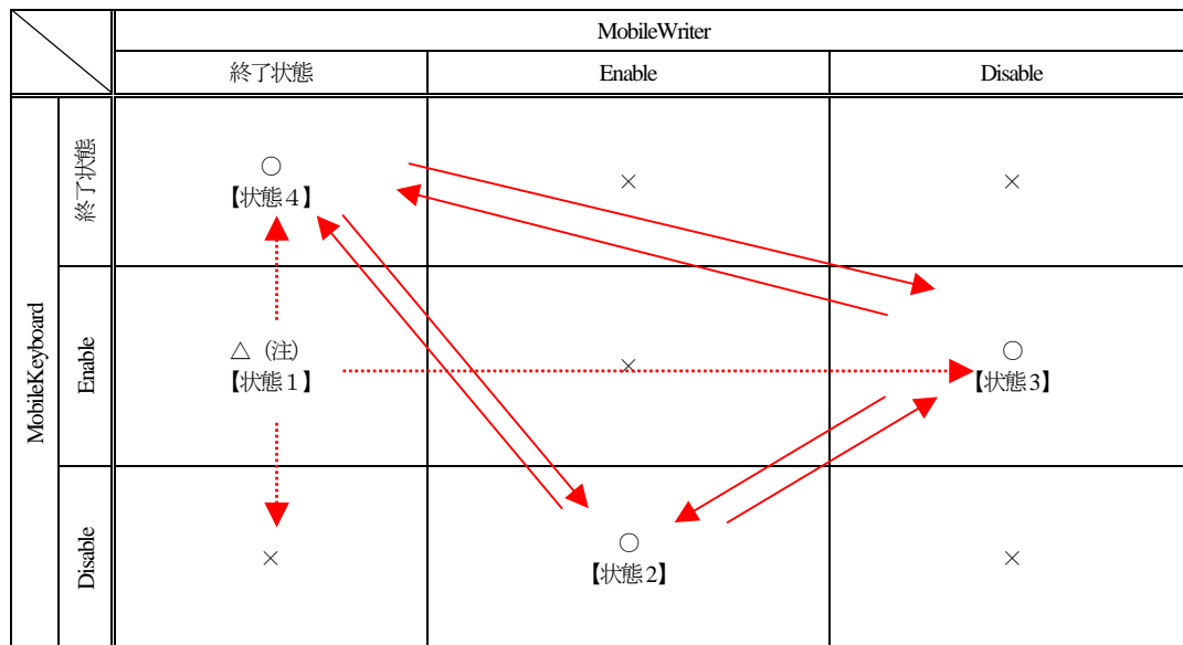
図3 状態遷移図
