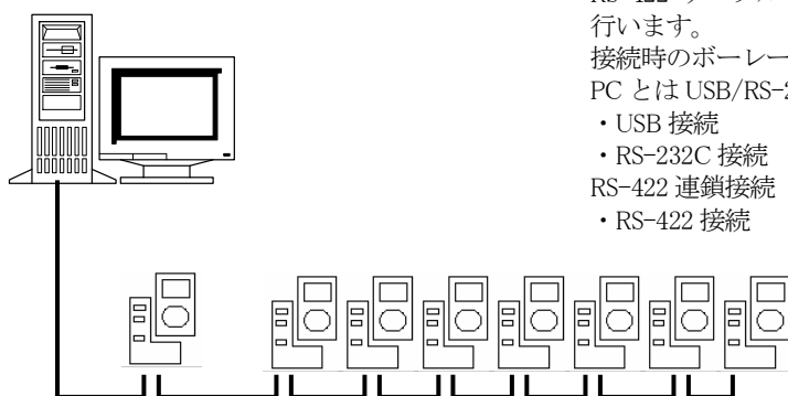
RS-422 連鎖接続
